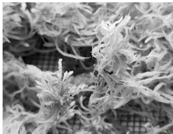
Природный сорбент, изучение поверхности под микроскопом, увеличение в 40 раз. Фото: пресс-служба ПетрГУ
